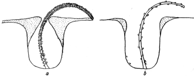
Fig. 1. Auf dem Pronotum gelegene Grube von a) Neides tipularius L., b) N. favosus Fieb. im Längsschnitt. Wachsschicht punktiert
