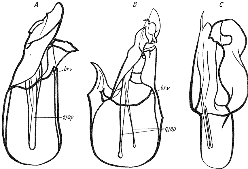
Fig 10. Hypandrium, dorsal, von Platypalpus striola OLDBG (A), Platypalpus ciliaris FALL (B), Platypalpus nigratarsis FALL (C)
